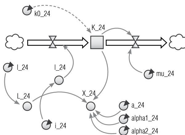
Рис. 1. Потоквая диаграмма металлургической отрасли
